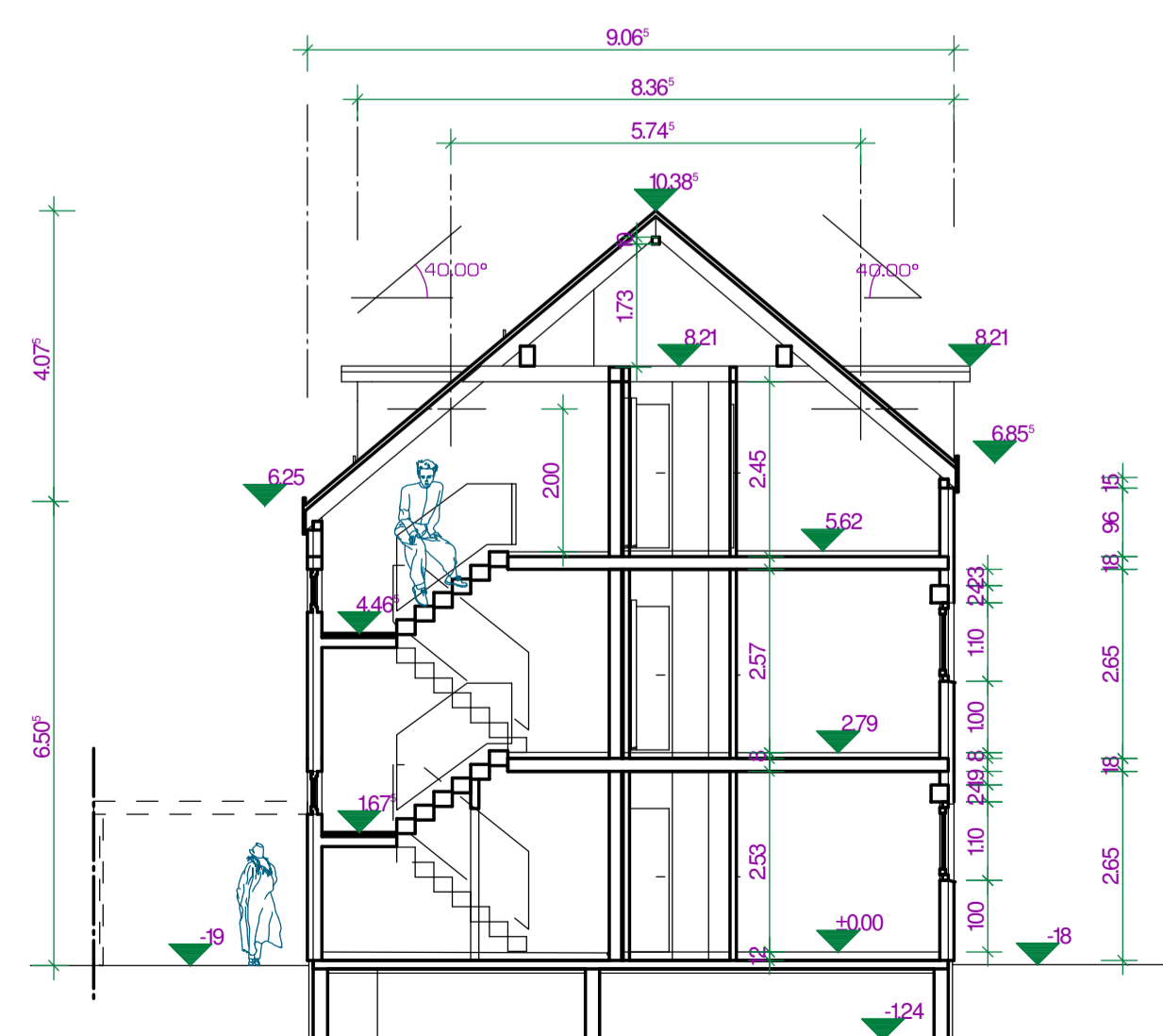
Schnitt A-A
