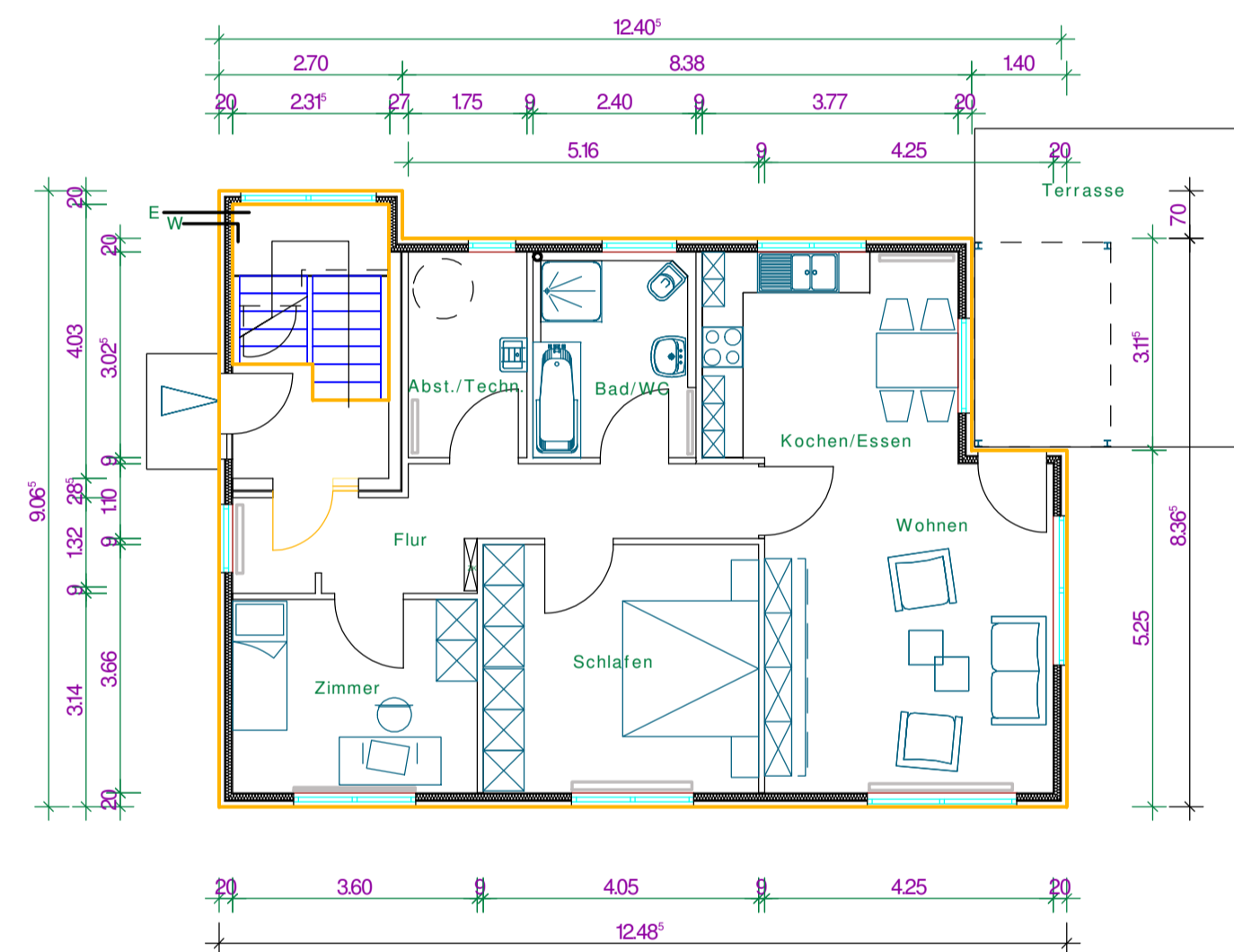
Erdgeschoss (Obergeschoss)
