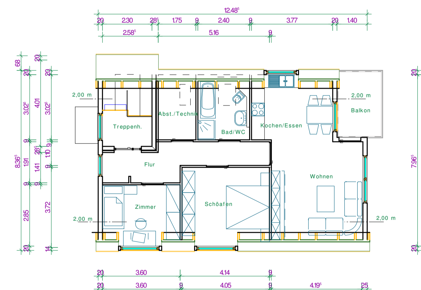
Dachgeschoss
