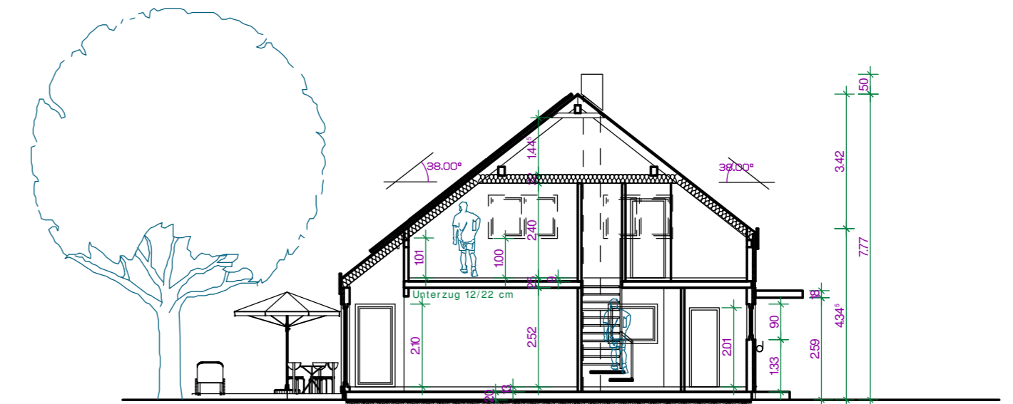
Schnitt A-A
