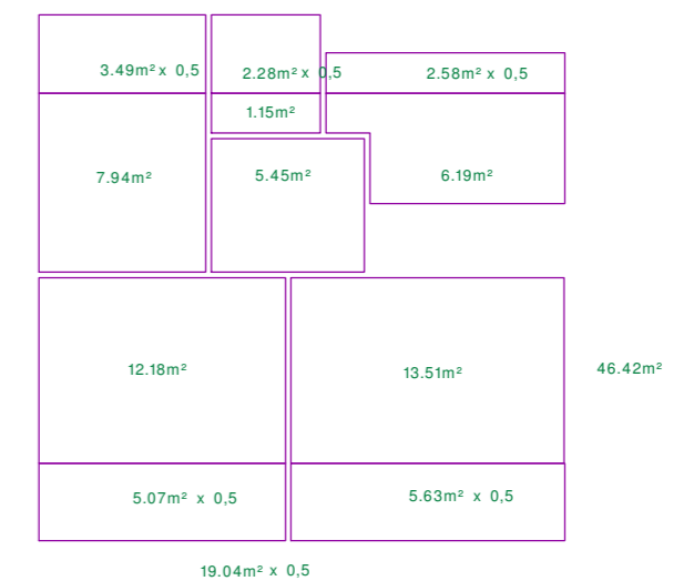
Haus: Bayern-Kompakt 136
